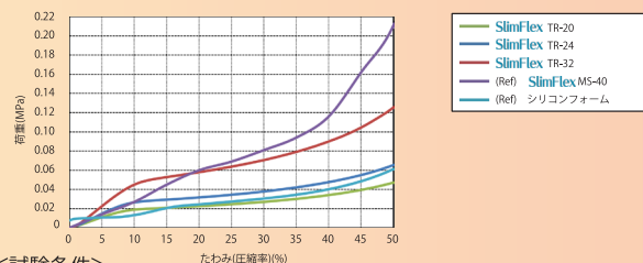
◆荷重-たわみ曲線
