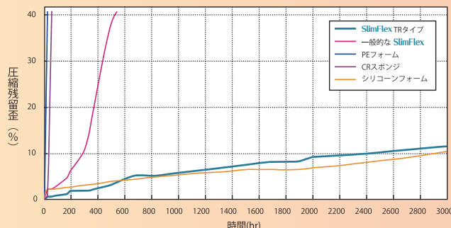
◆圧縮残留歪 (長期連続圧縮)
